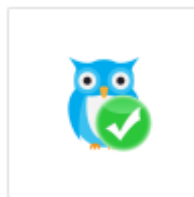
ChkEliteXOT.exe
